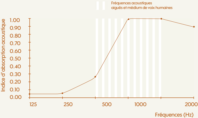
Courbe du coefficient d'absorption acoustique pratique conformément à la norme NF EN ISO 354
